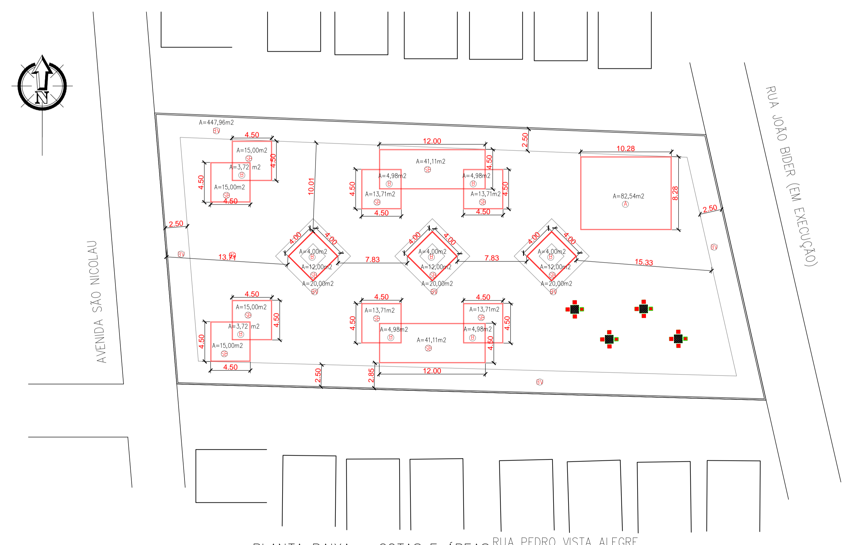
PLANTA BAIXA – COTAS E ÁREAS ESCALA 1/250 RUA PEDRO VISTA ALEGRE
