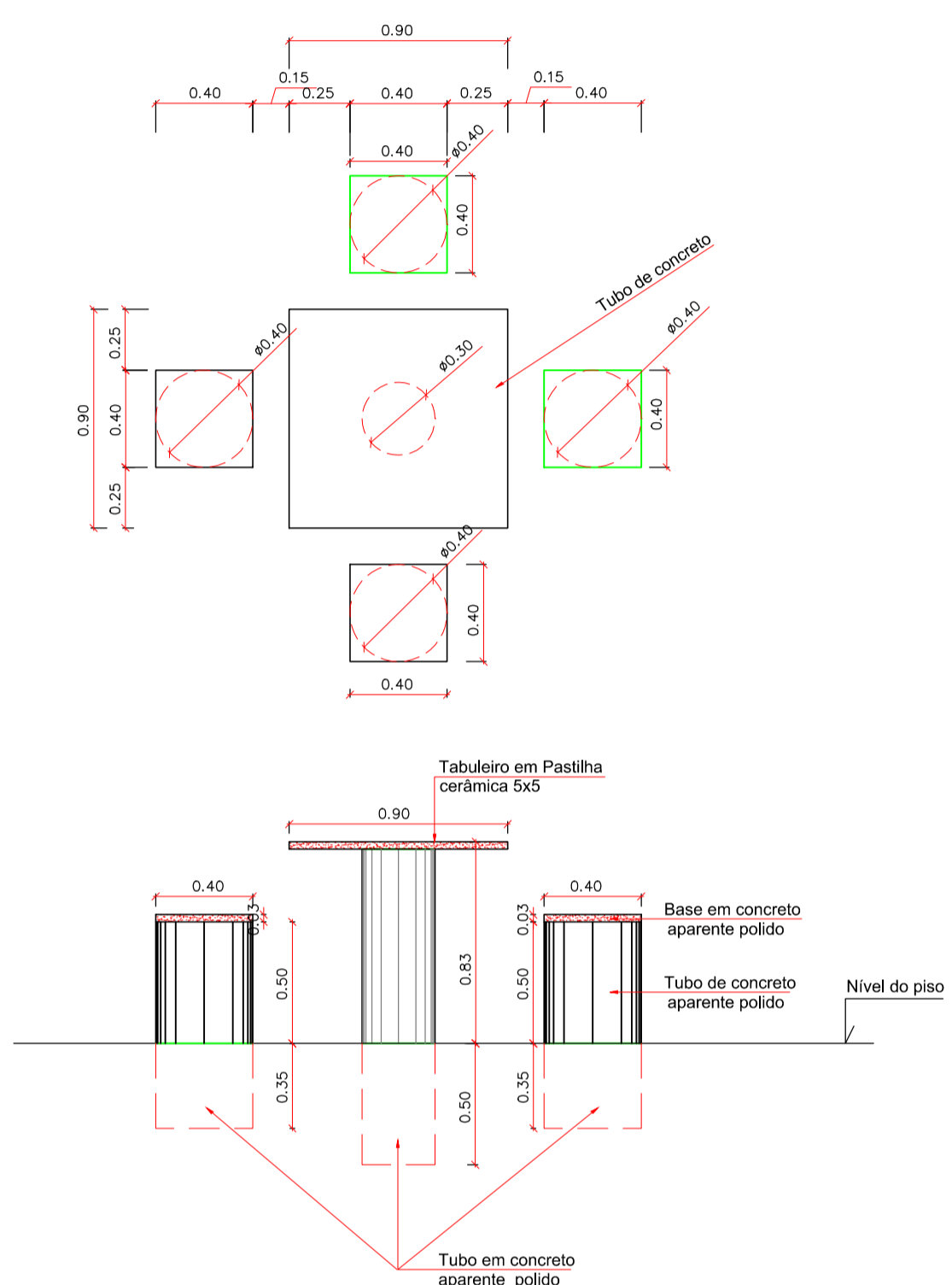
MESA DE CONCRETO / BANCO EM TUBO DE CONCRETO ESCALA 1/25
