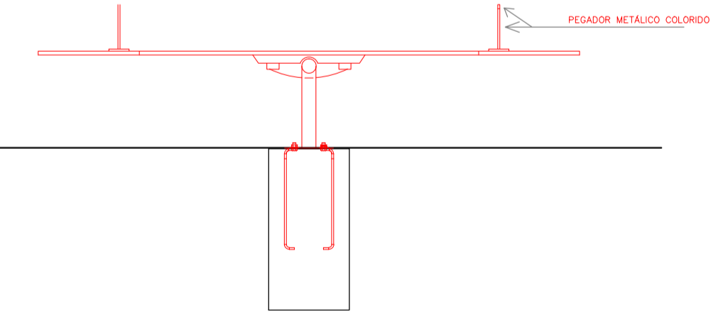
VISTA LATERAL- BRINQUEDO 02 esc 1:25
