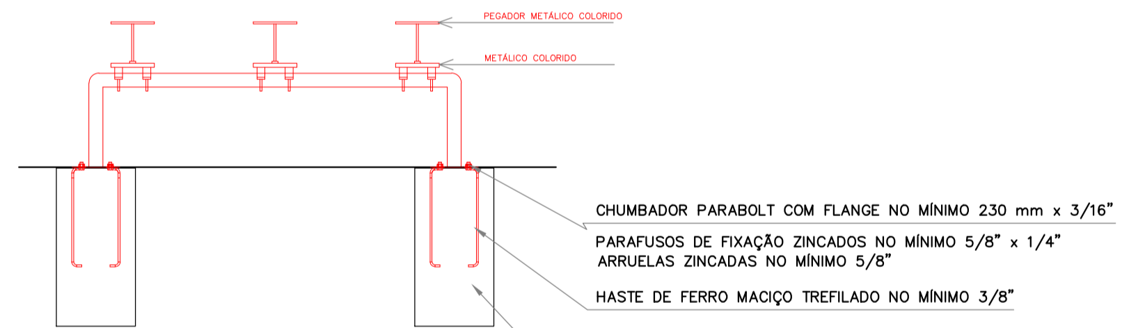
VISTA FRONTAL- BRINQUEDO 02 esc 1:25
